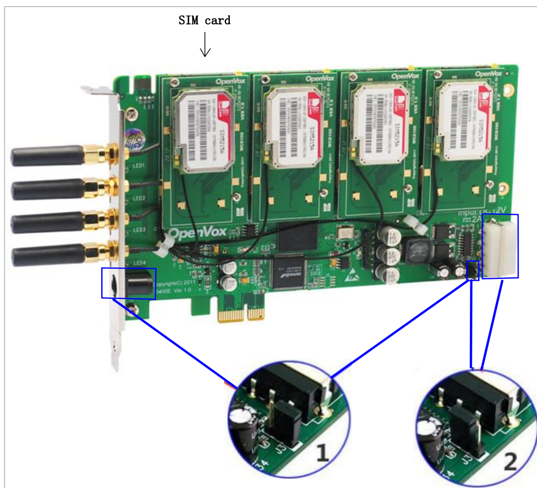
图 3 两种供电方式
