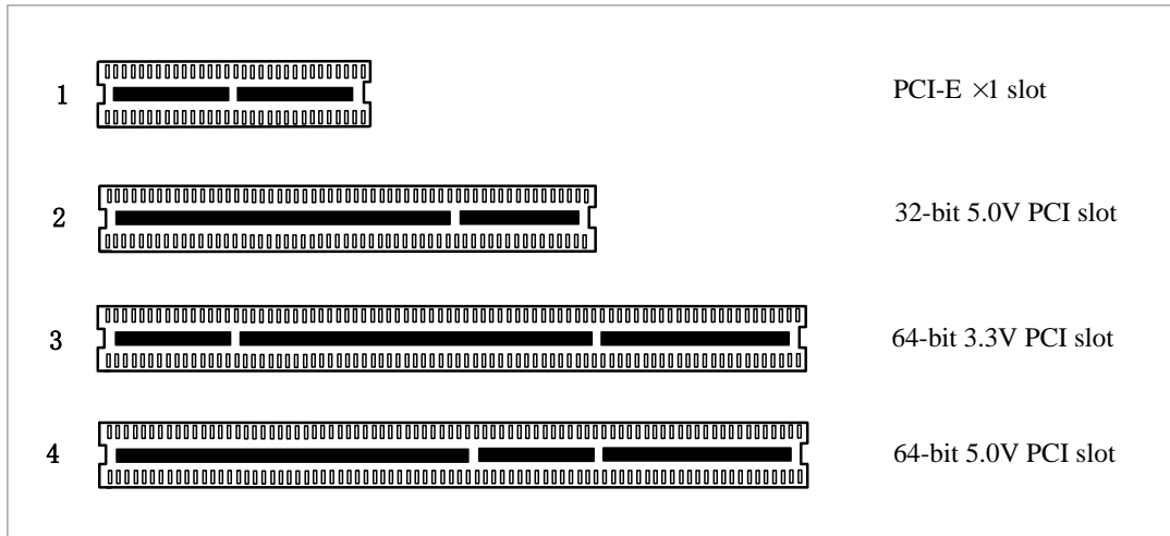
图2 PCI及PCI-E插槽
