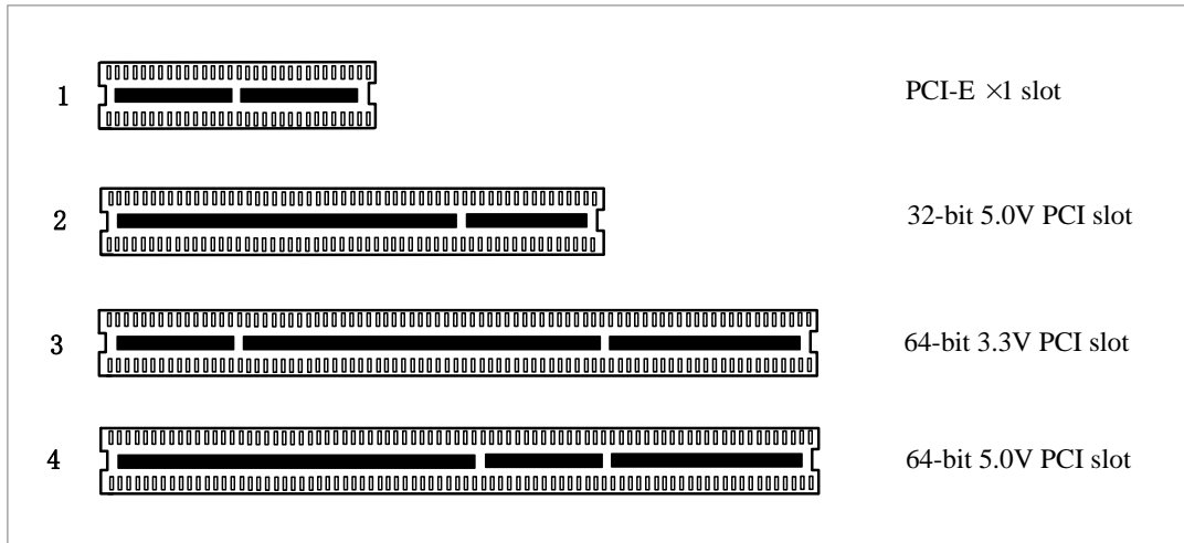
图2 PCI及PCI-E插槽
