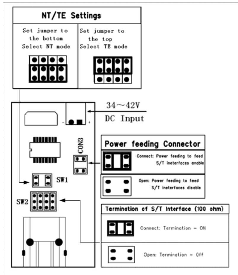
图 3 B100M跳线设置
