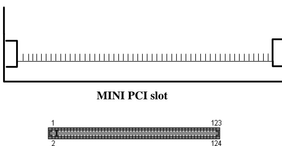
图 2 124针的迷你PCI III型 (AMP 1318228-1) 连接器
