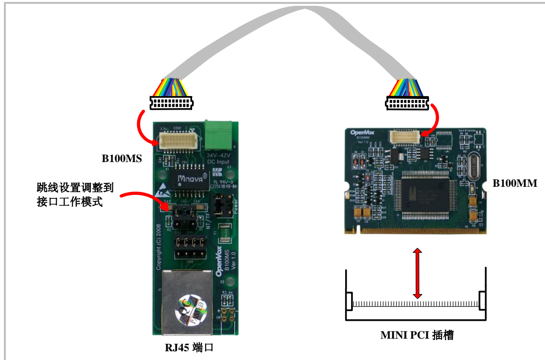
图 4 连接线
