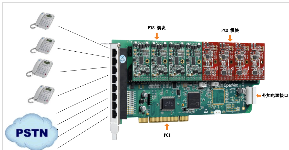
图 2 典型应用
