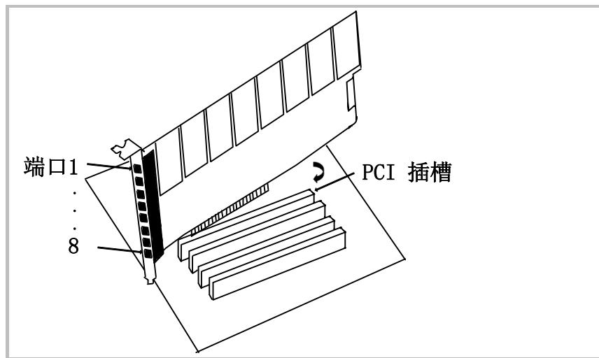
图4 硬件安装
