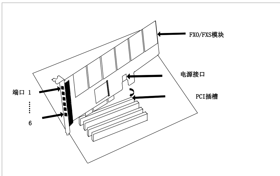
图3 硬件安装
