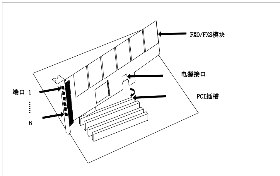
图3 硬件安装
