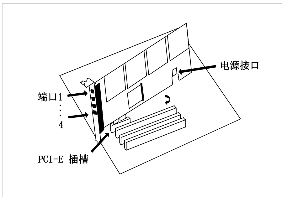
图4 硬件安装
